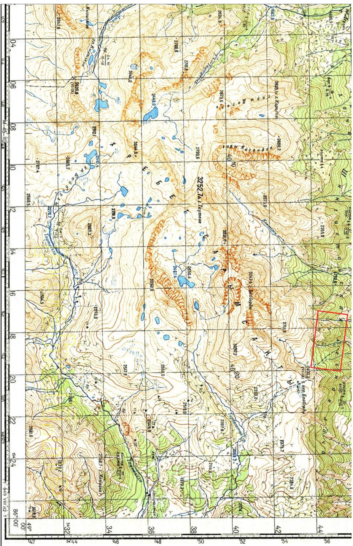
1-сызба. Сарымсақты жотасының топографиялық картасы
