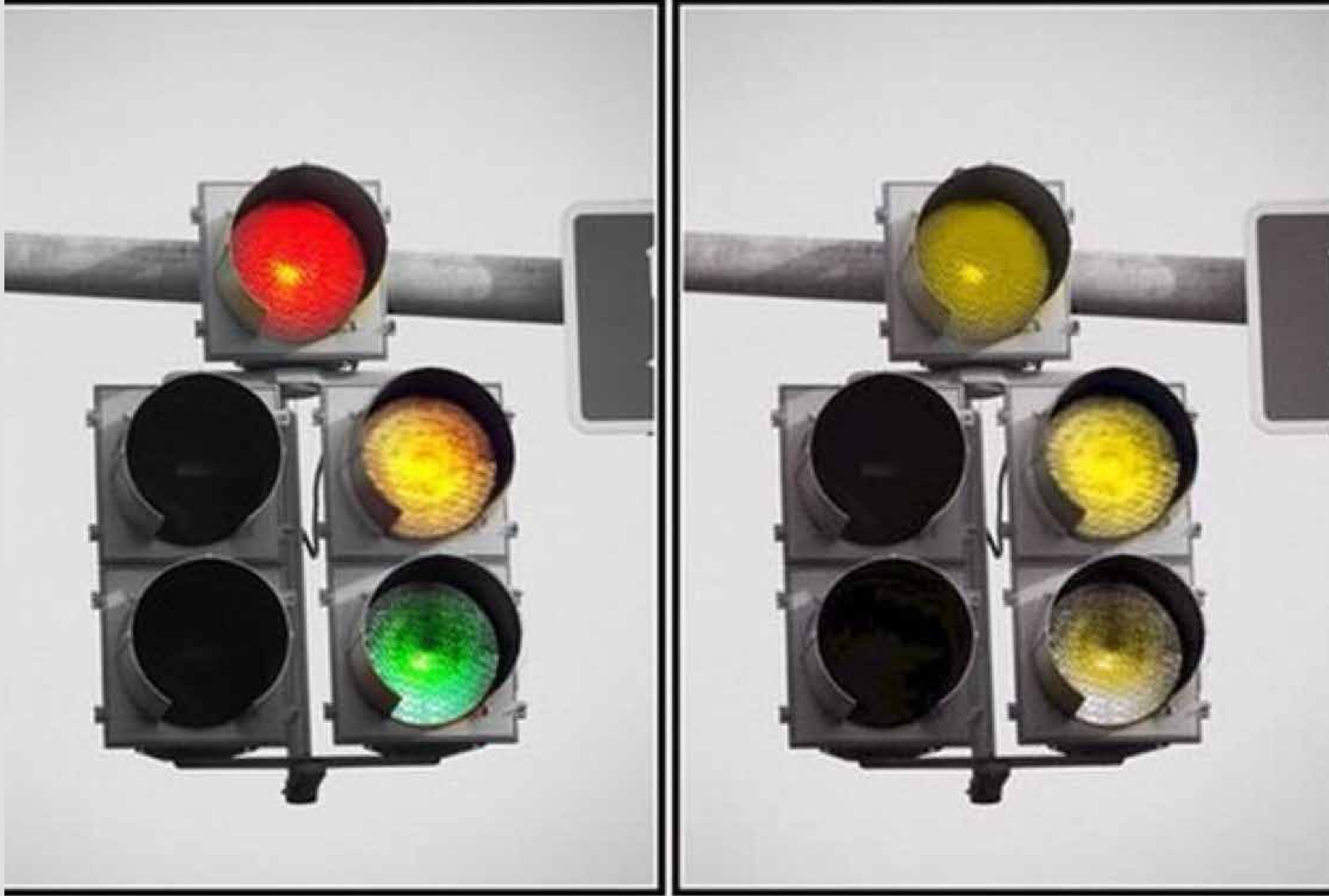
Как видят светофор: с нормальным зрением (слева) и с дальтонизмом (справа)
